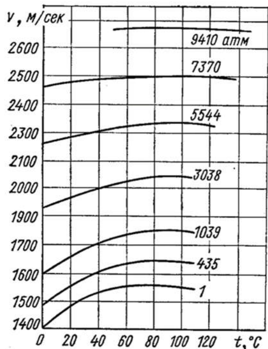
Зависимость скорости ультразвука (частота 12 МГц) в воде от давления и температуры
